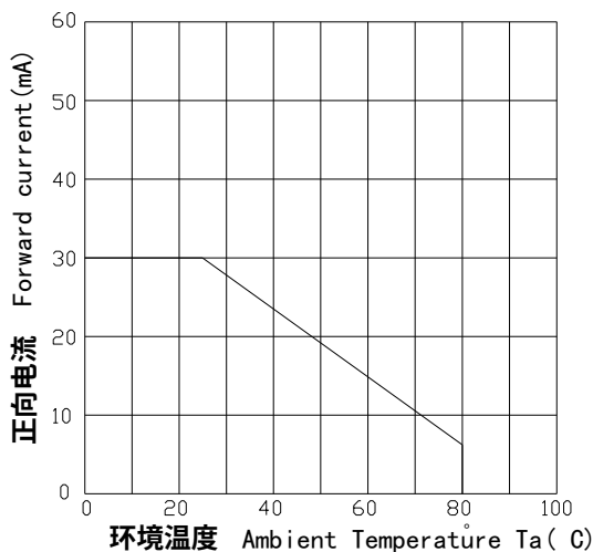
正向电流额定参数曲线
